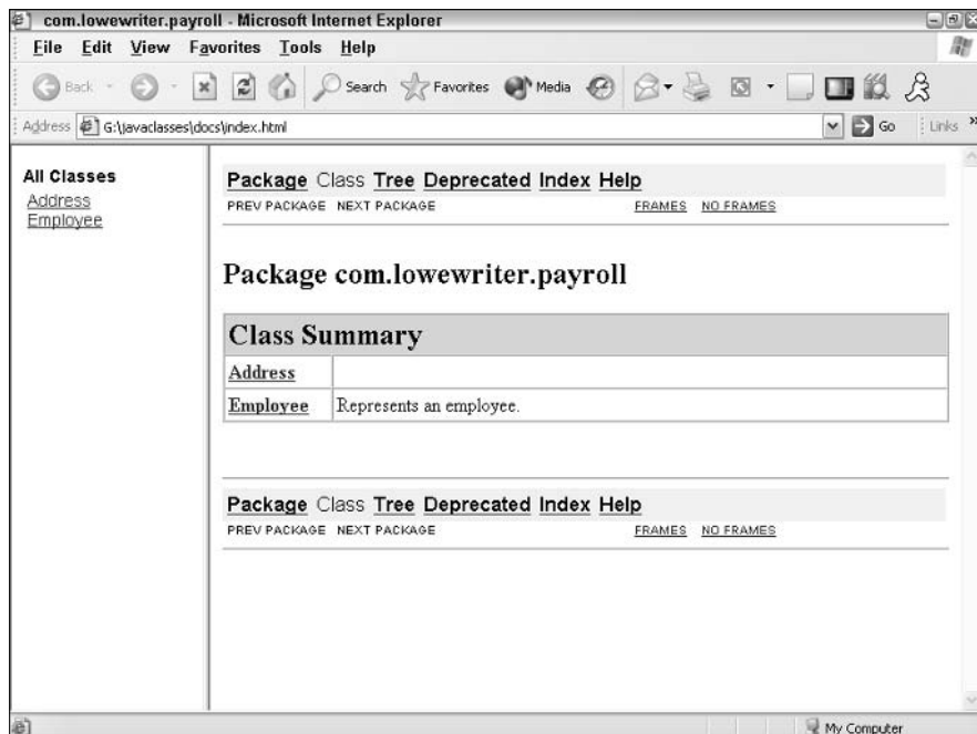
Figure 8-1: A JavaDocs index page.
