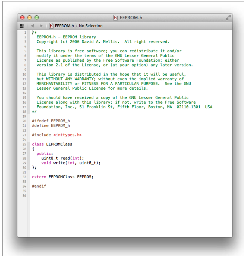
EEPROM.h displayed in Xcode IDE
