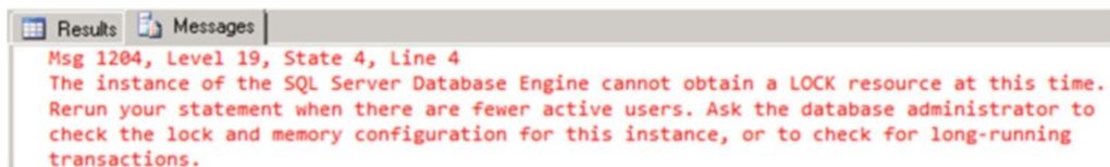
Figure 20-8. Error 1204
