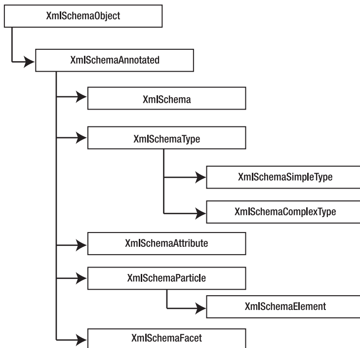
Figure 5-11. The SOM object hierarchy
