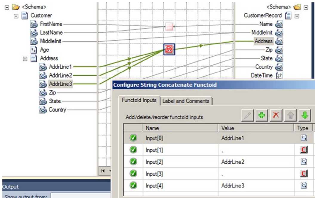
Figure 3-6. String concatenation mappings
