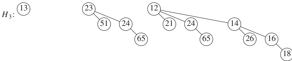
Figure 6.46 Binomial queue H_3
