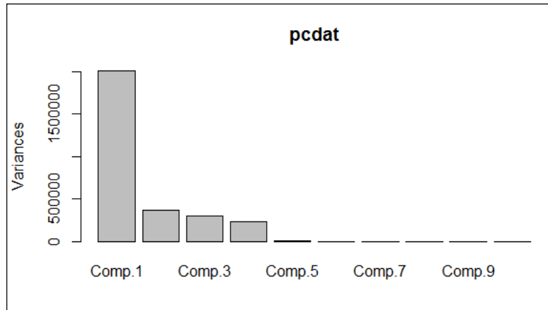
PCA output
